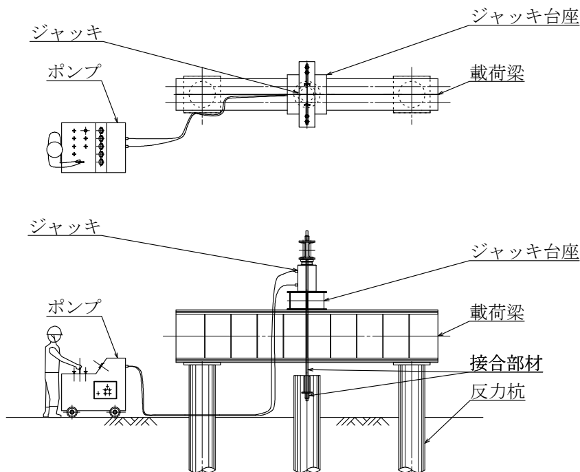
図6—載荷装置の例（反力抵抗体として反力杭を用いる場合）
