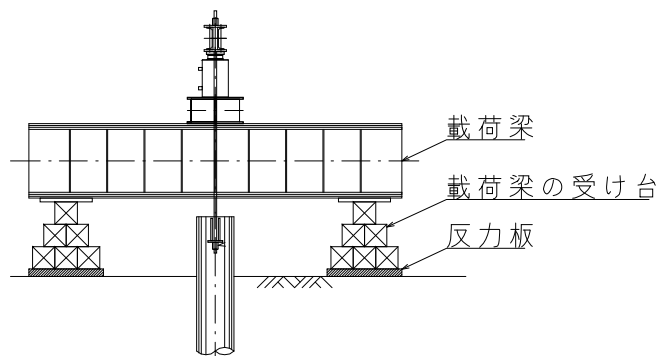
図7—反力板を用いる場合の載荷梁の支持形式の例
