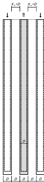
a) 試験杭に拡径部がない場合
