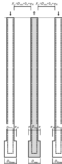
b) 試験杭に拡径部がある場合
